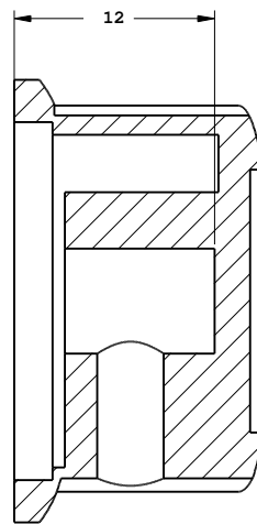
Schnitt A-A
